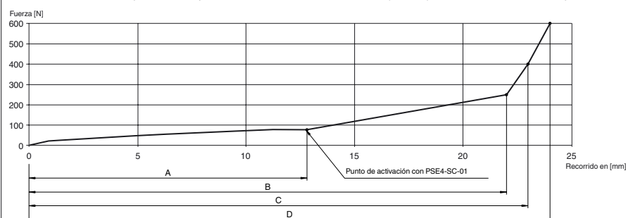
Diagrama del recorrido de la fuerza Parámetros de medición: T = 23 °C, posición de montaje B conforme a EN 1760-2, ubicación de medición C (EN 1760-2), v = 100 mm/s hasta A, v = 10 mm/s a partir de A.
